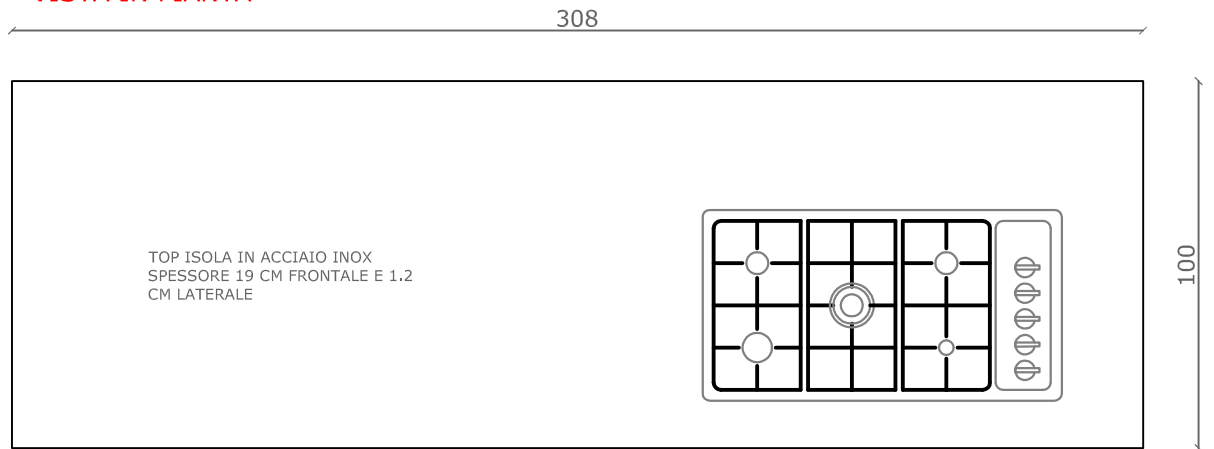
BLOCCO ISOLA VISTA IN PIANTA
