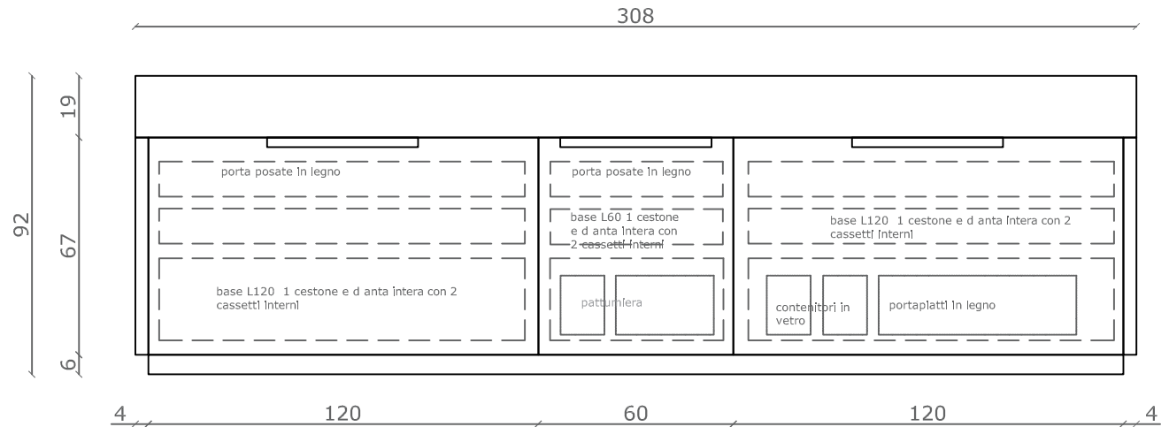
BLOCCO ISOLA VISTA LATO 2
