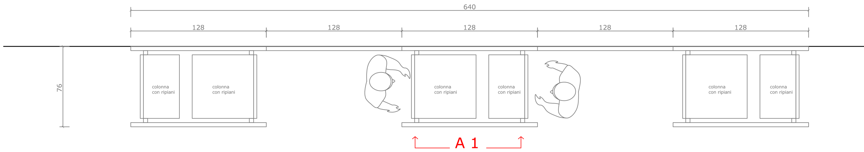
vista planimetrica
