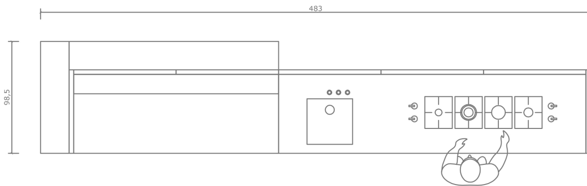
pianta
